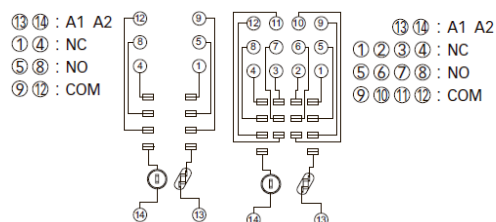
Схема соединений
