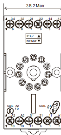
KS-B 3CO Размеры (мм)
