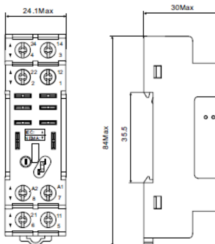
KS-R 2CO Размеры (мм)
