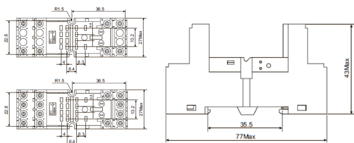
Размеры KS 2CO / KS 4CO (мм)
