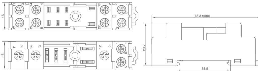
Размеры KRI 1CO / KRI 2CO (мм)
