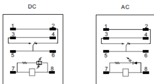
KRL100 Схема подключения
