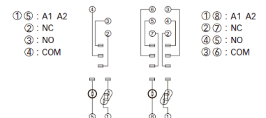
Схема соединений
