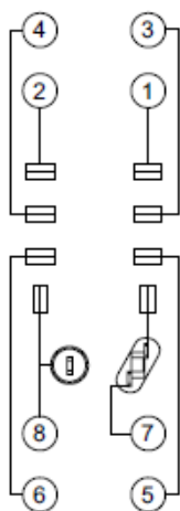
KS-R 2CO Схема соединений
