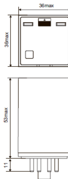
KRB300 Размеры, мм
