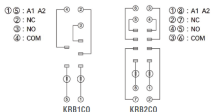
Схема соединений
