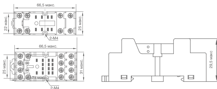
Размеры KS 2CO ECO / KS 4CO ECO (мм)
