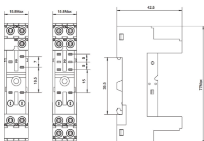
Размеры KRI 1CO / KRI 2CO (мм)
