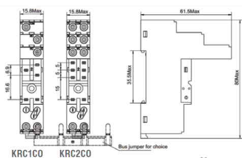
Размеры KRC 1CO / KRC 2CO (мм)
