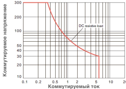
KRM400 Отключающая способность
