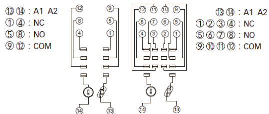
Схема соединений
