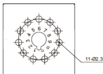
KRB300 Схема подключения
