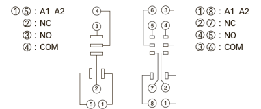
Схема соединений
