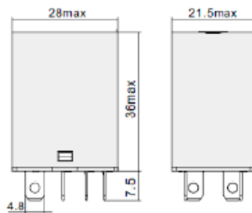
KRL100 Размеры (мм)
