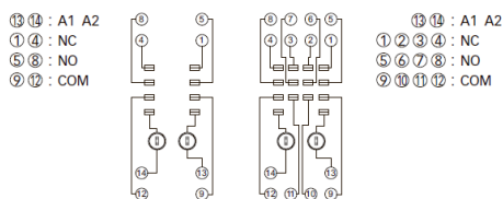
Схема соединений
