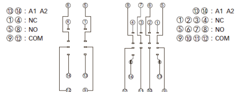
Схема соединений
