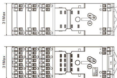
Размеры KS-C-ST 2CO / KS-C-ST 4CO (мм)
