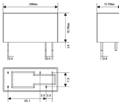
KRG100 Размеры (мм)
