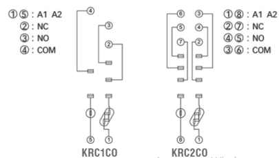
Схема соединений
