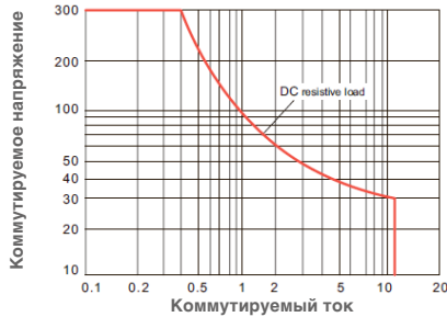
KRM200 Отключающая способность
