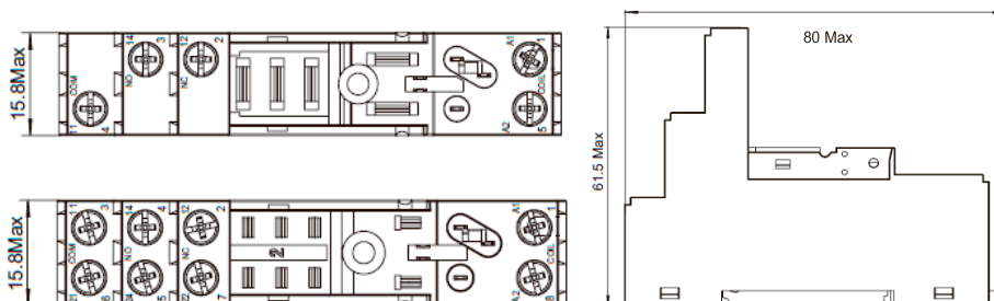
Размеры KRI 1CO / KRI 2CO (мм)
