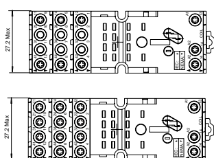
Размеры KS-C 2CO / KS-C 4CO (мм)
